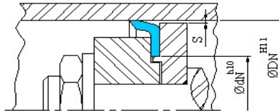
Vedação do Êmbolo
