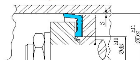
Vedação do Êmbolo
